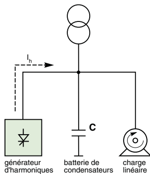
Schéma réel d'une installation.
